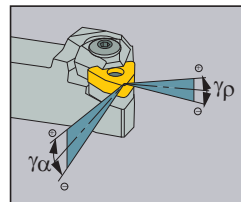
Державка наружная
